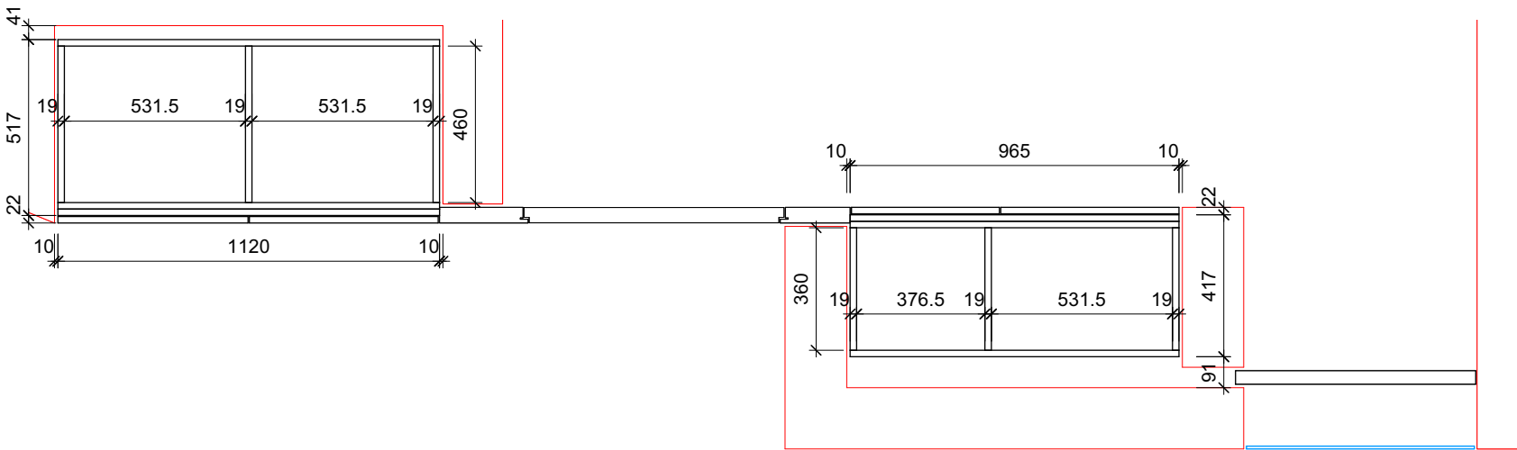
B-B Sockelplan
